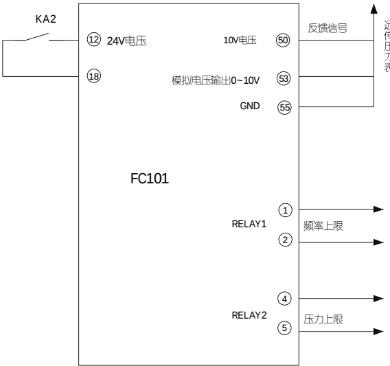
FC101接线图
