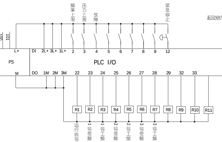
PLC接线图
